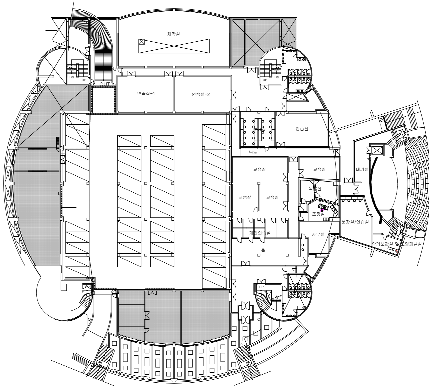
지하1층 평면도
