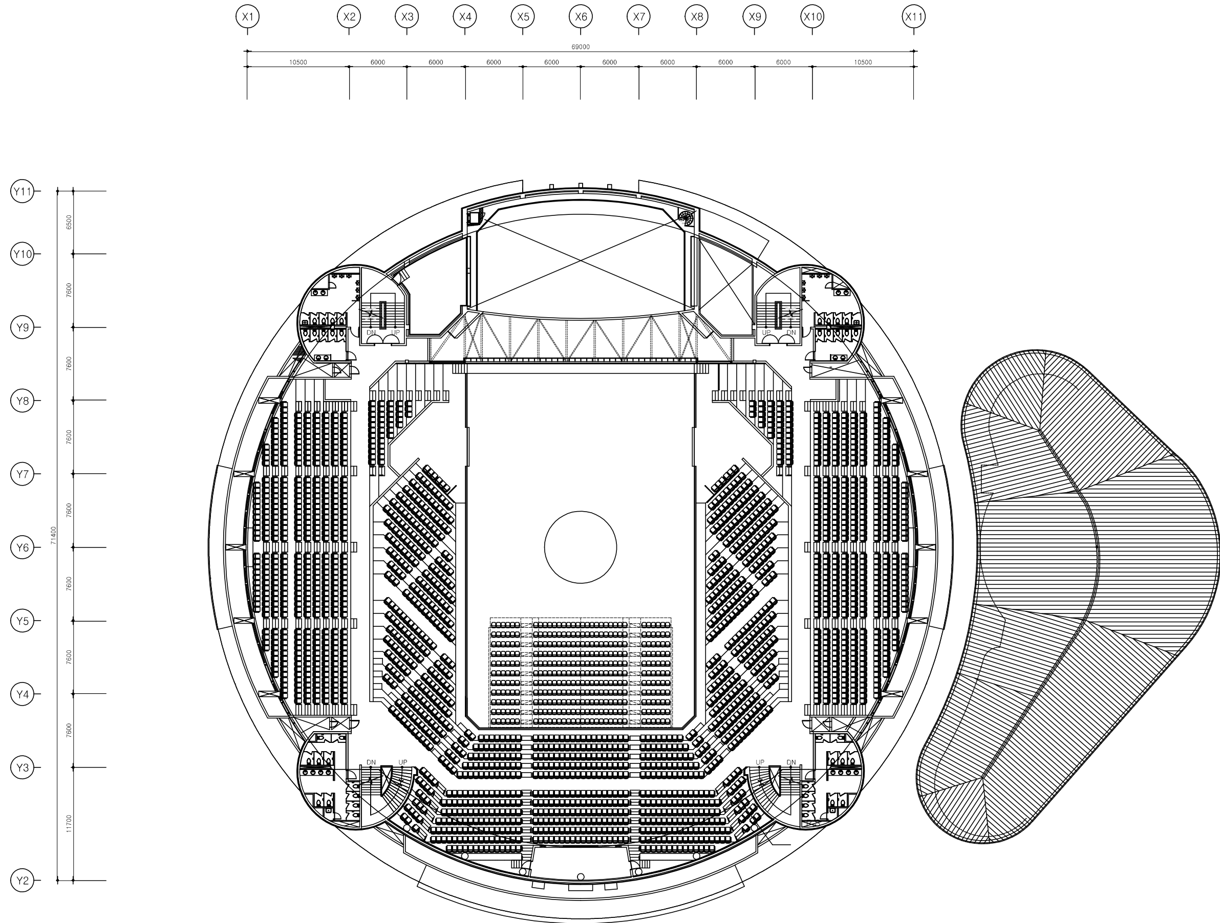
지상2층 평면도
